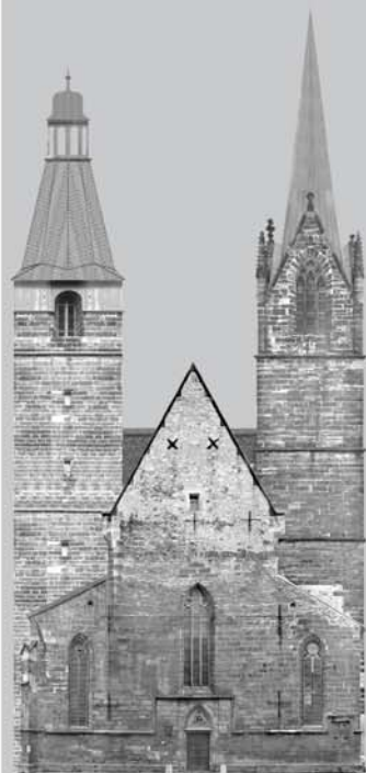
Ansicht von Westen - Bestand
